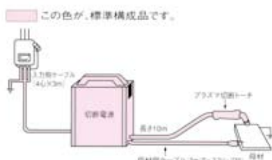
【M5500C II 接続図】
