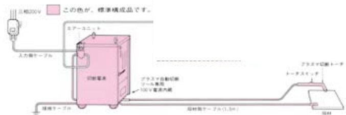
【D-8000, D-12000 接続図】
